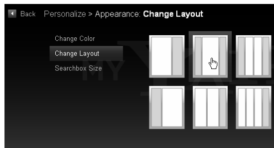
Gambar 1.38 Pengaturan Layout
